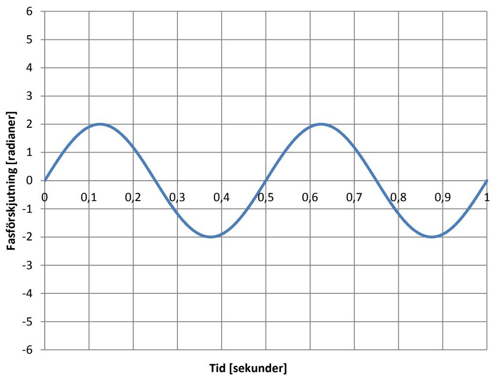
Fasförskjutningen \Theta(t)
